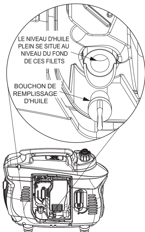
Figure 9 - Remplissage d'huile
